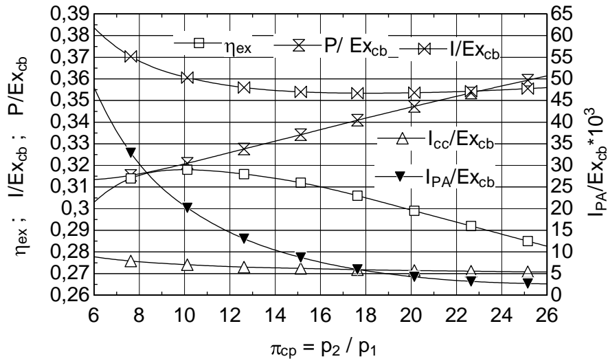
Figure 6 : Influence du rapport de compression sur le rendement exégétique et sur les destructions et pertes relatives d'exergie de l'installation turbine à gaz avec échangeur récupérateur de préchauffage de l'air ( \theta = 5 , \eta_{PA} = 0,75 , G_a = 25 \text{ kg}/(\text{m}^2 \text{ s}) , G_g = 12 \text{ kg}/(\text{m}^2 \text{ s}) )
